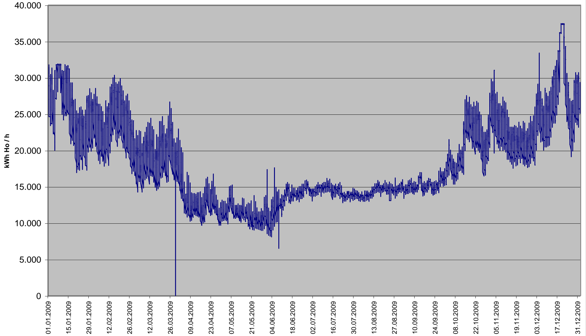
Lastgang Bezug SWW [ kWh Ho / h ]
