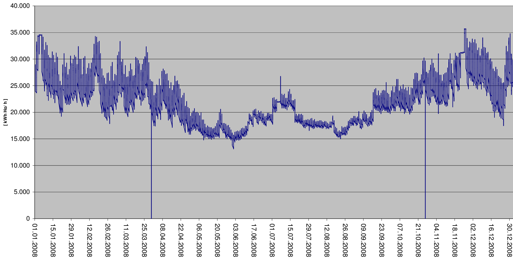
Lastgang Stadtwerke Weißwasser GmbH 2008 [ kWh Ho ]
